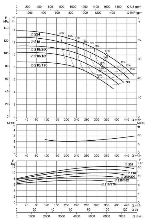
KDN 150-200
