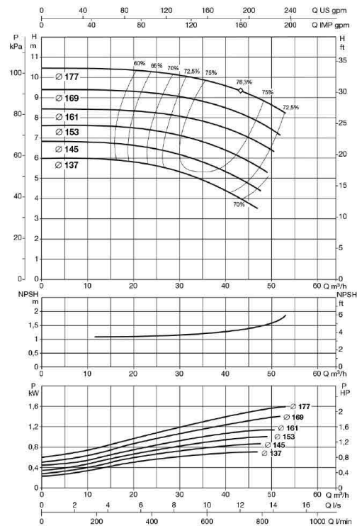
KDN 50-160
