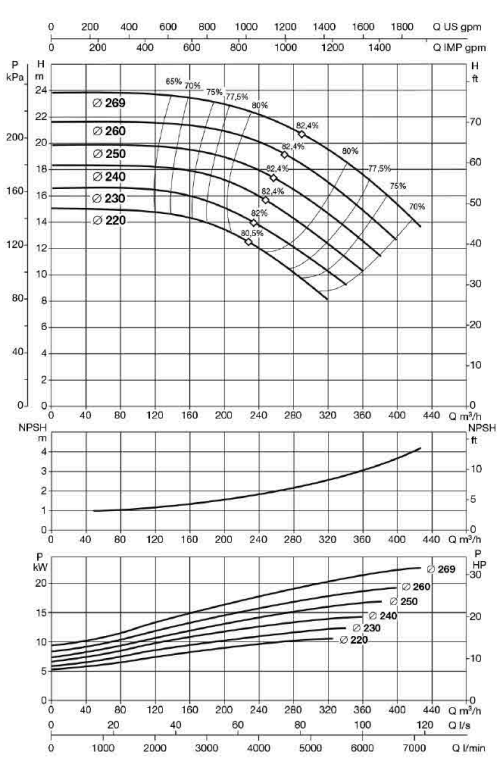
KDN 125-250
