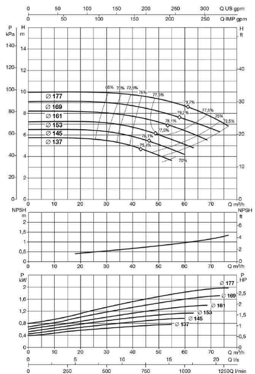
KDN 60-160
