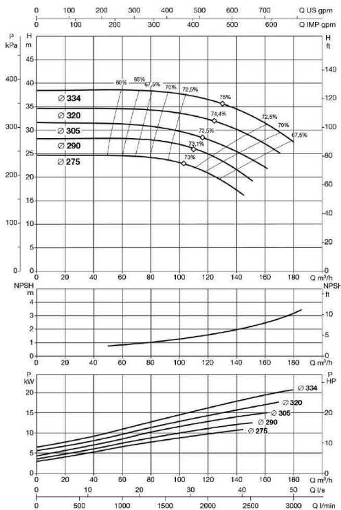
KDN 80-315
