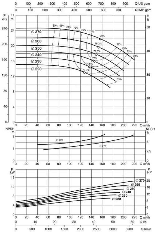
KDN 100-250
