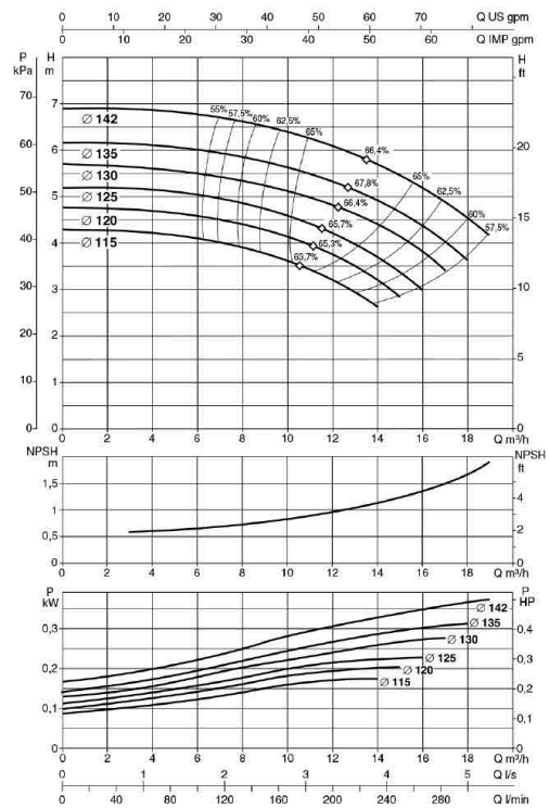
KDN 32-160
