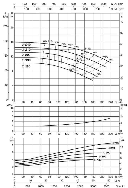
KDN 100-200
