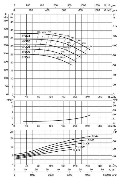
KDN 150-200
