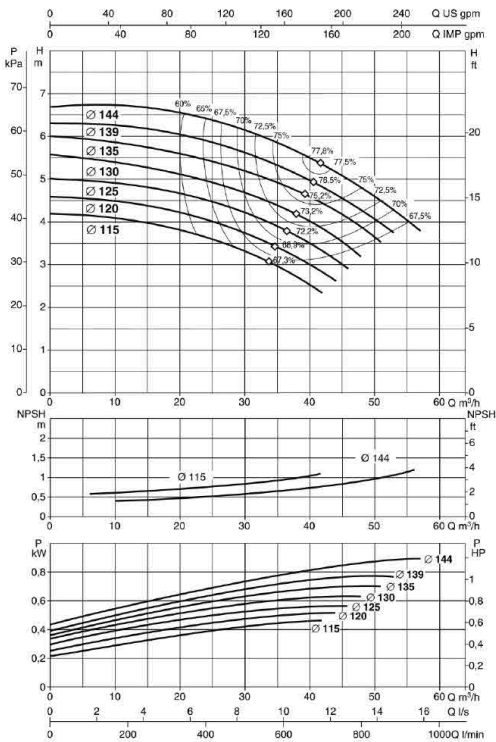
KDN 50-125
